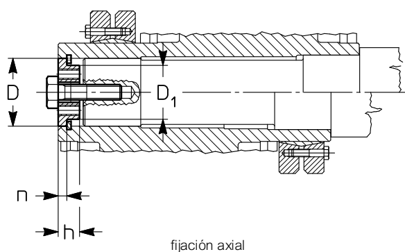
fijación axial
