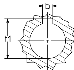
Árbol (hueco) máquina
