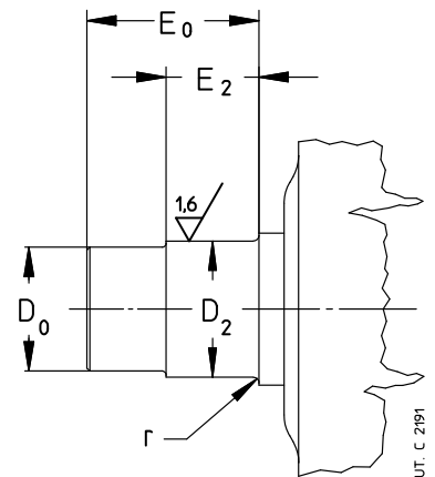
(b) Perno de máquina «corto» (excluidos tam. 7101, 8001)
