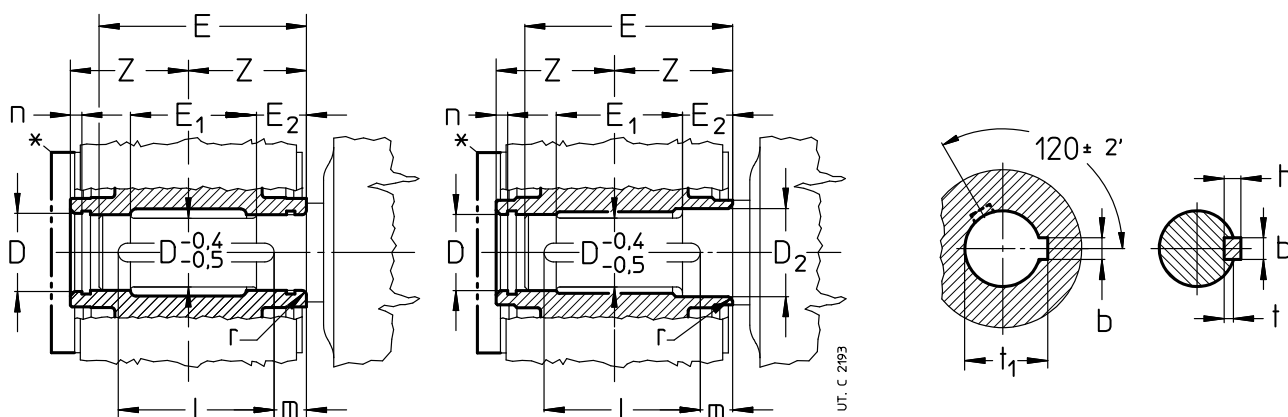
(a) Árbol lento hueco con chavetero
