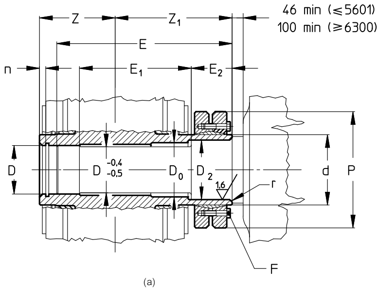
(a) Árbol lento hueco diferenciado con unidad de bloqueo y perno de máquina «largo»
